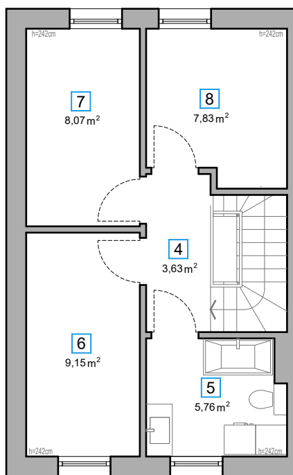
RZUT Poddasza
