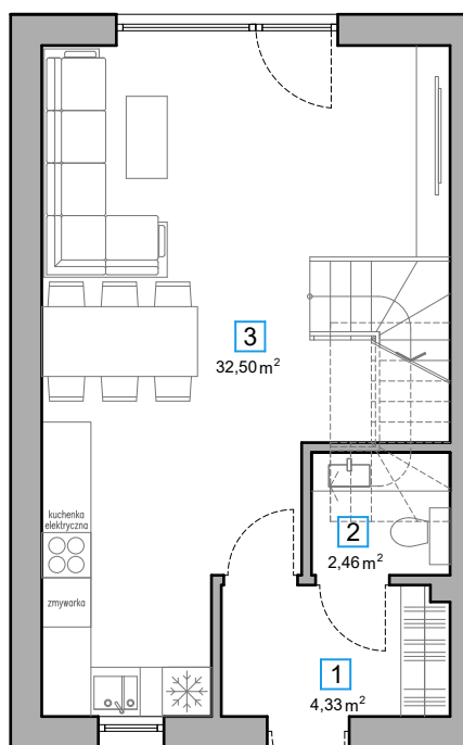
RZUT PARTERU
