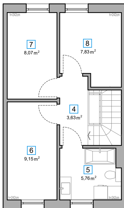
RZUT PODDASZA
