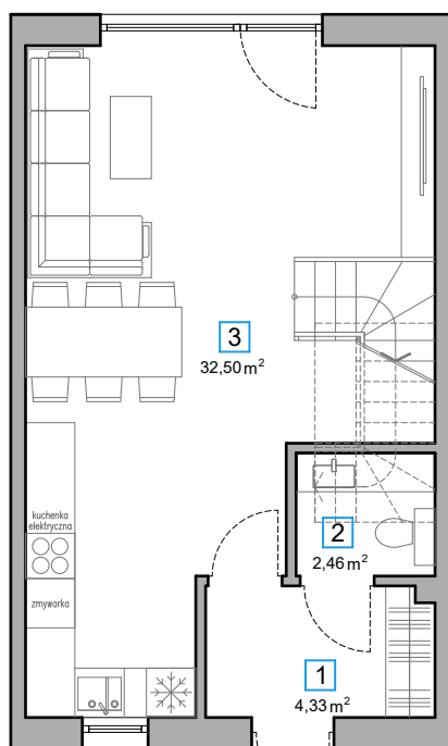
RZUT PARTERU
