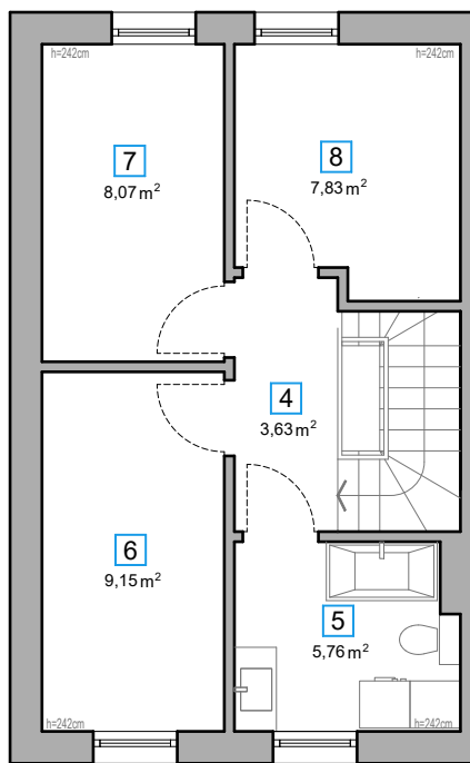
RZUT PODDASZA 34,44 m 2
