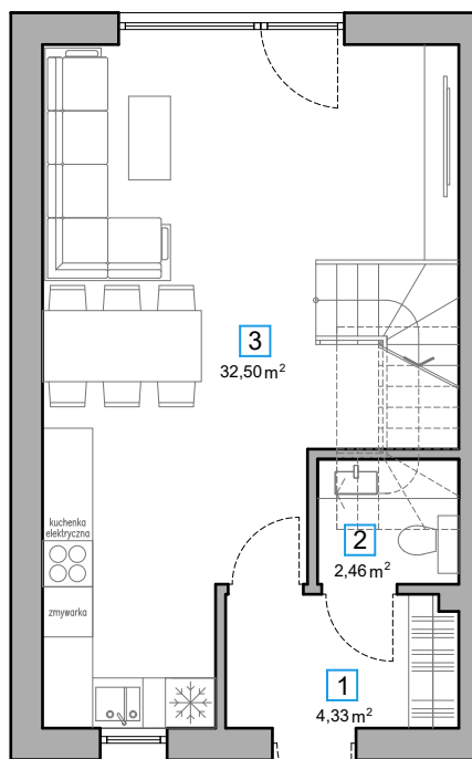
RZUT PARTERU 39,29 m 2
