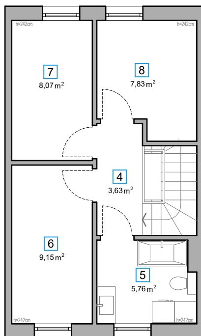
RZUT PODDASZA
